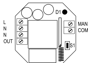
Rys. 1 Widok sterownika
